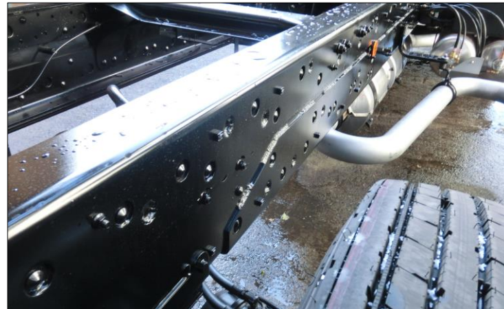
施工例D
