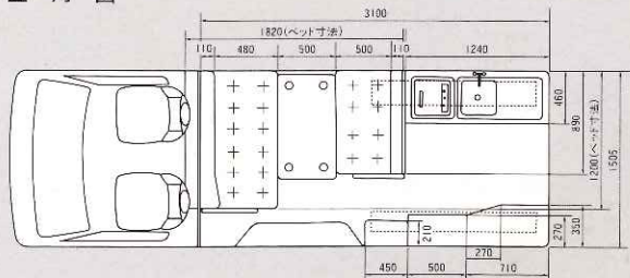
室内図
