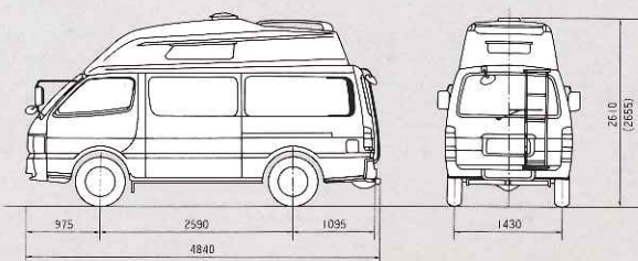
外観寸法図
