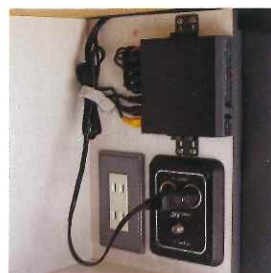
■ダイバーシティユニット(オプション) AC・DCコンセント
