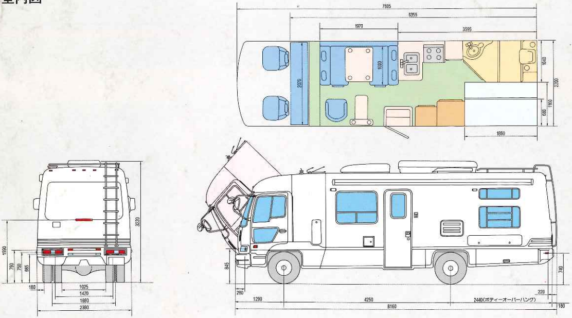
外観 & 室内図
