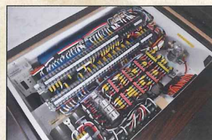
■ 電装盤
